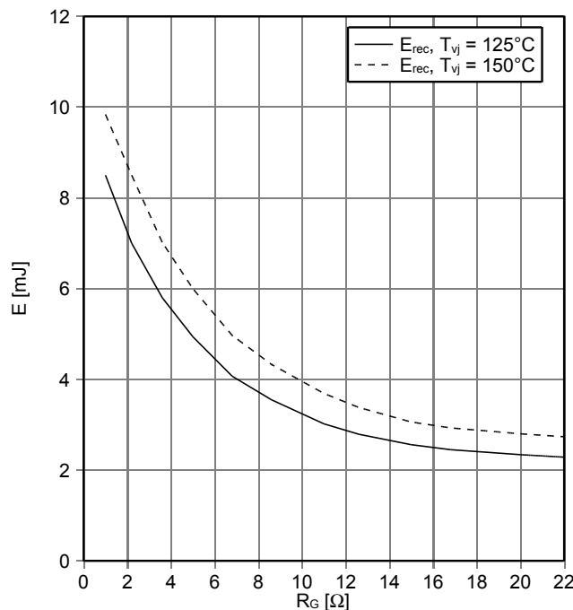
Schaltverluste Diode, Wechselrichter (typisch) switching losses Diode, Inverter (typical) E_{rec} = f(R_G) I_F = 400 A, V_{CE} = 300 V
