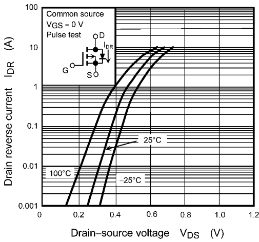
Fig. 7.9 I_{DR} - V_{DS}
